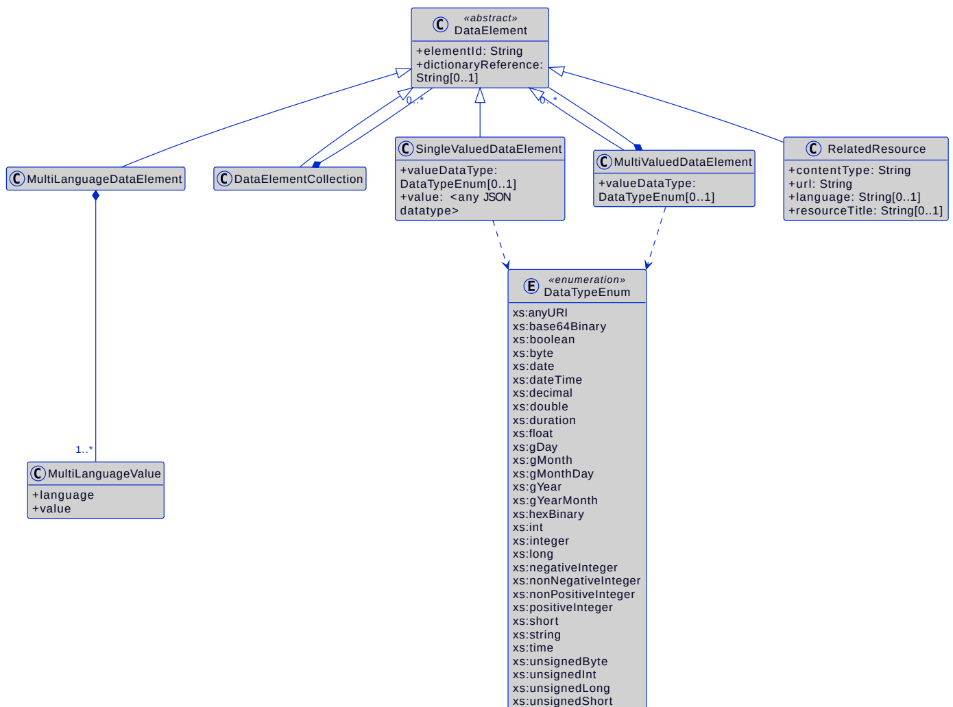
Figure 66. Overview metamodel for data points (EN 18223)
